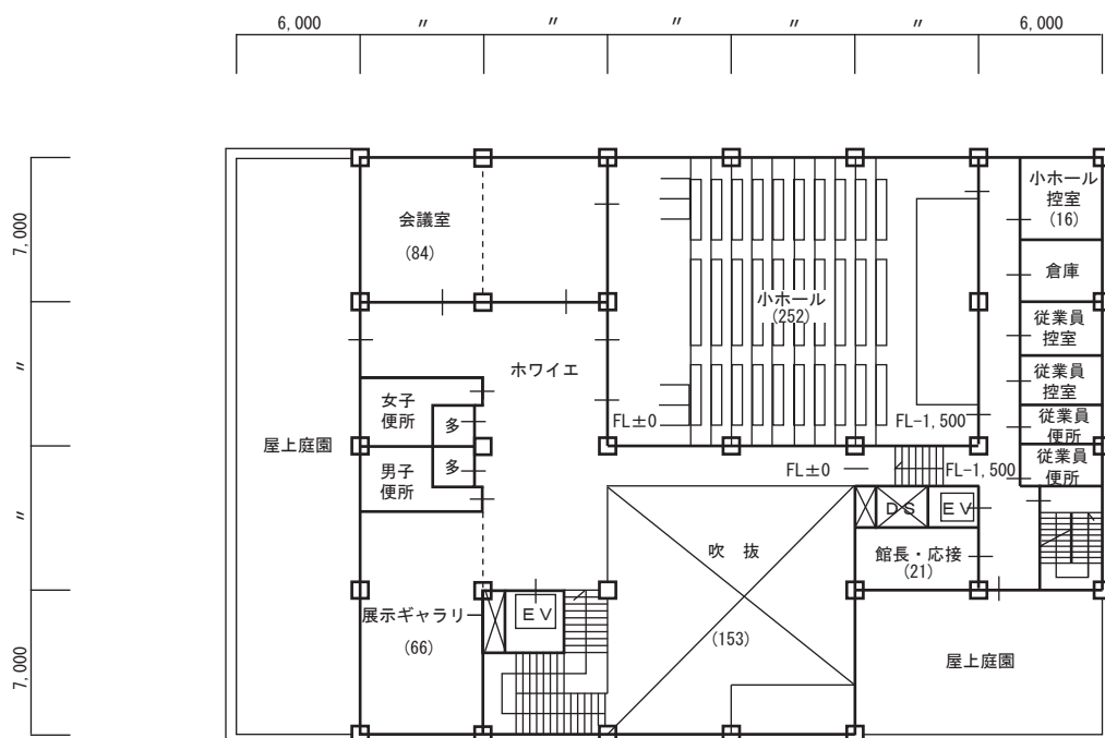
2 階平面図 1/400
