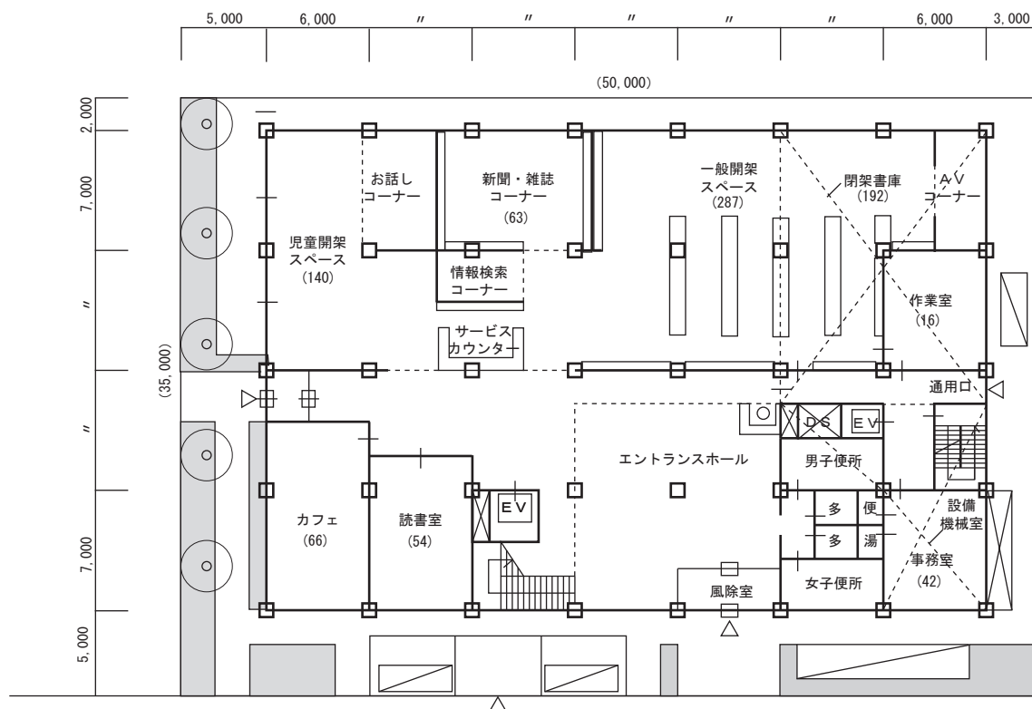
1 階平面図兼配置図 1/400
