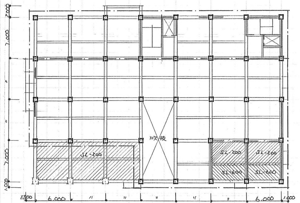
2階梁伏
