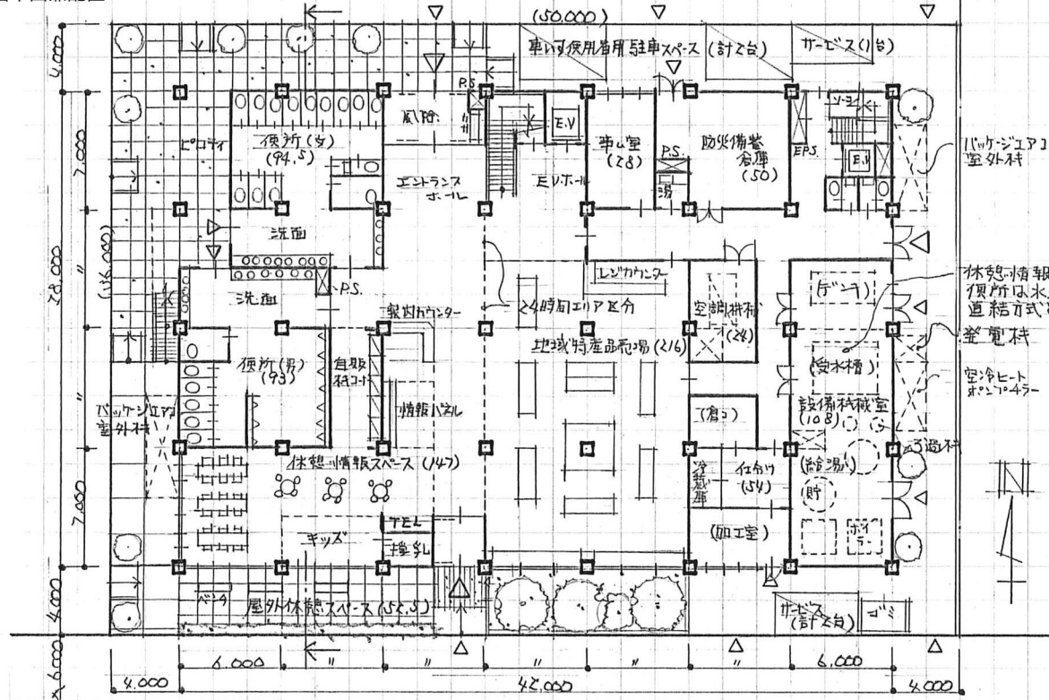
1階平面兼配置
