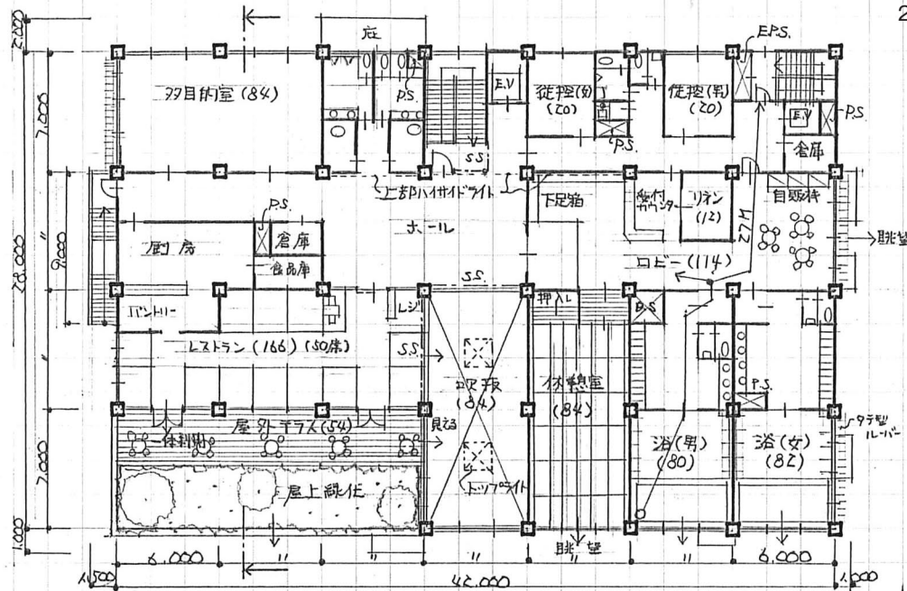
2階平面
