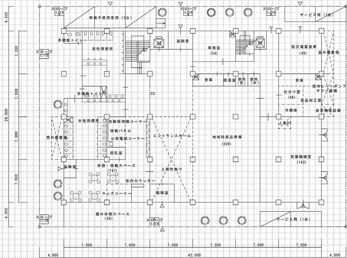
1 階平面図兼配置図
