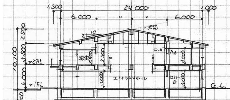
断面図 (S:1/400)
