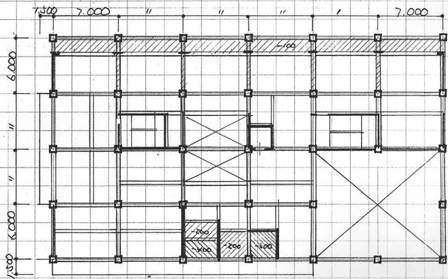
2階梁伏図 (S:1/400)
