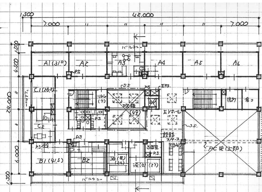
2階平面図 (S:1/400)
