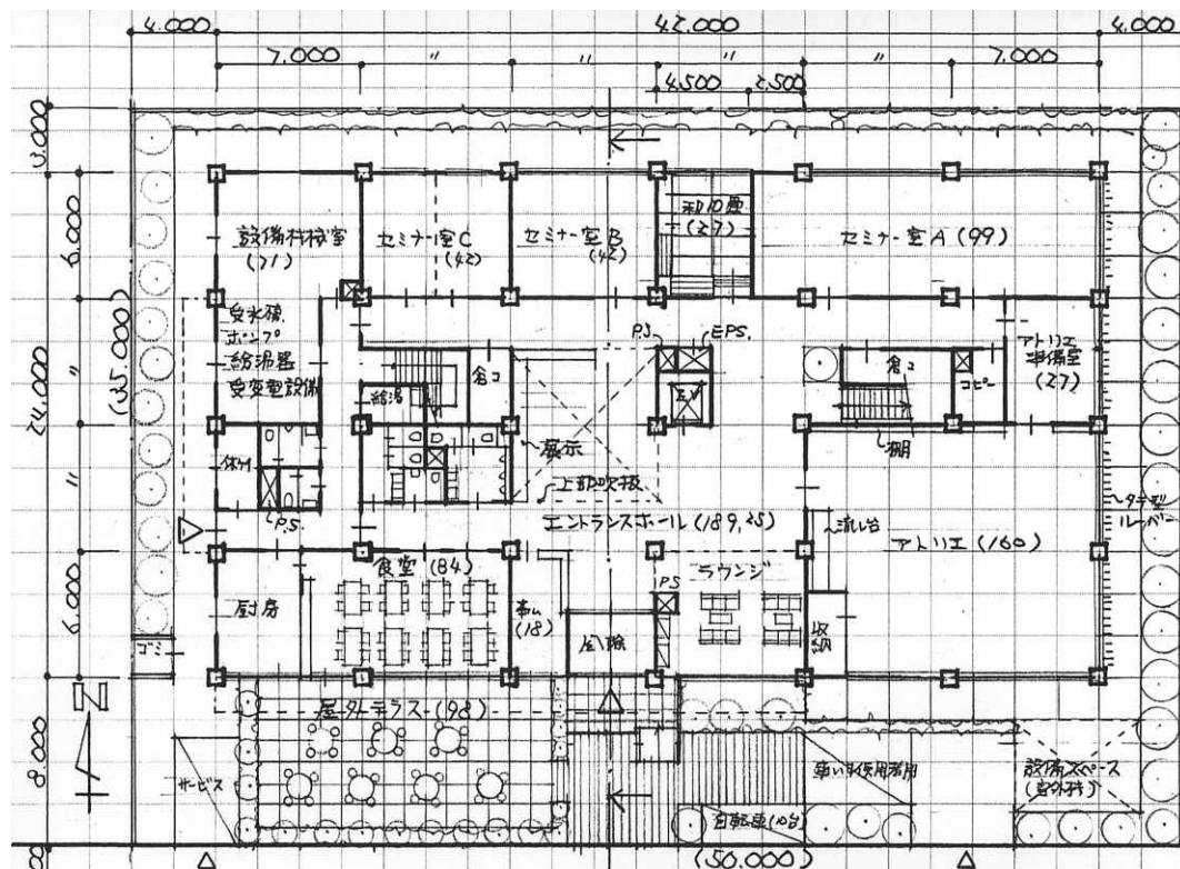
1階平面兼配置図 (S:1/400)
