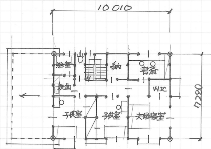
2階平面図
