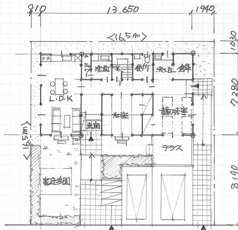
1階平面図
