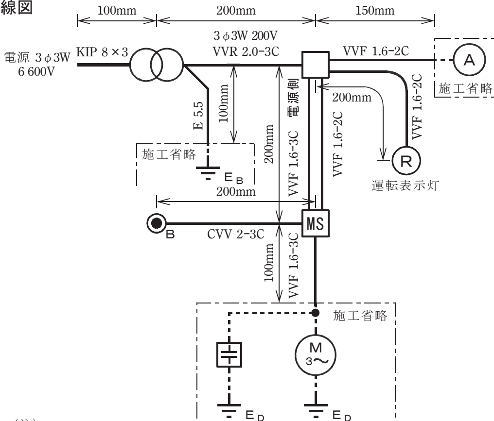
図 1. 配線図
